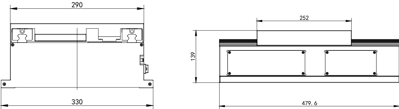
定子 +240mm 动子外形尺寸图
